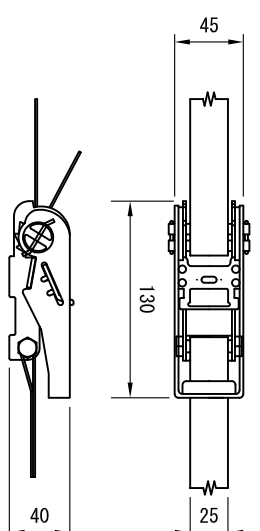
⑤ ライト付パイプ 1.5ton用2m S=1/5
