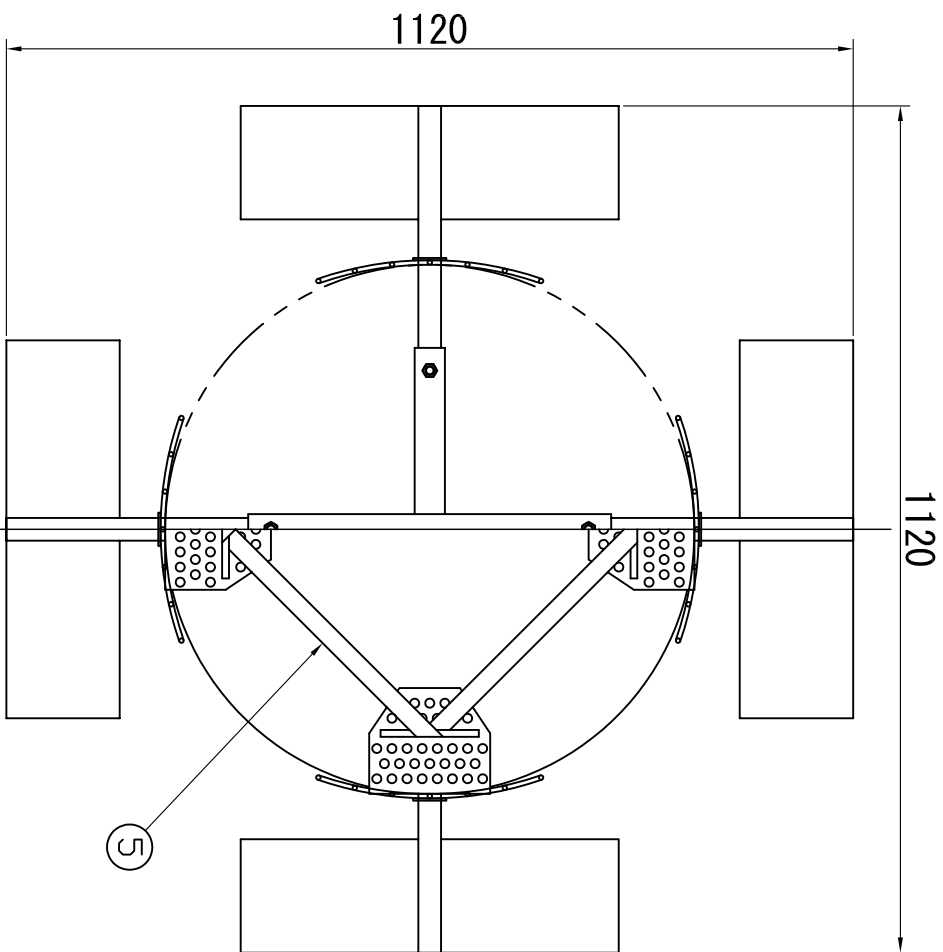
組図 S=1/10
