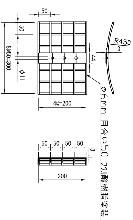
⑦ 根鉢側面押え 詳細図 S=1/10
