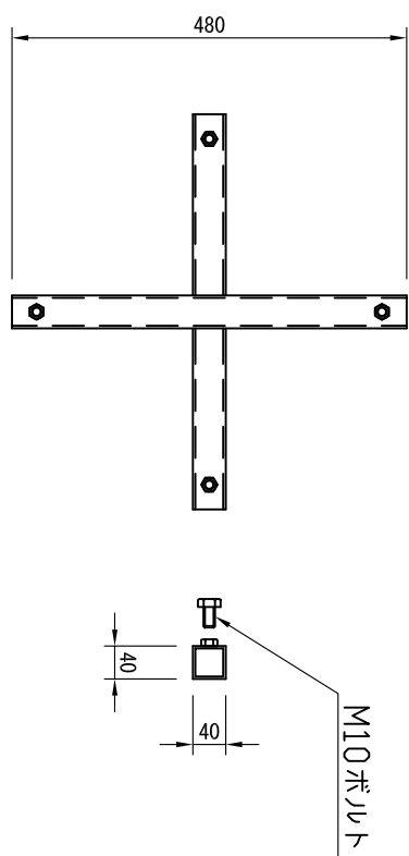
① 集合管 S=1/10
