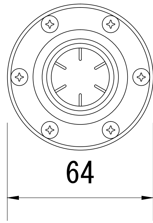
”A”-”A”矢視
