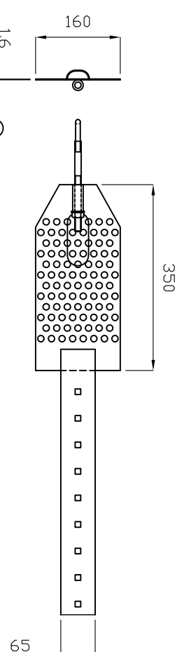
④ 固定板 S=1/10
