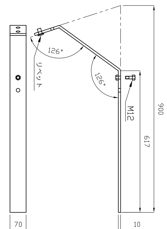
① 主板 S=1/10
