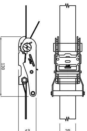
⑤ ライト付ハルト 2.0ton用5m S=1/5
