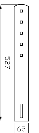
③ 連結金具 S=1/10
