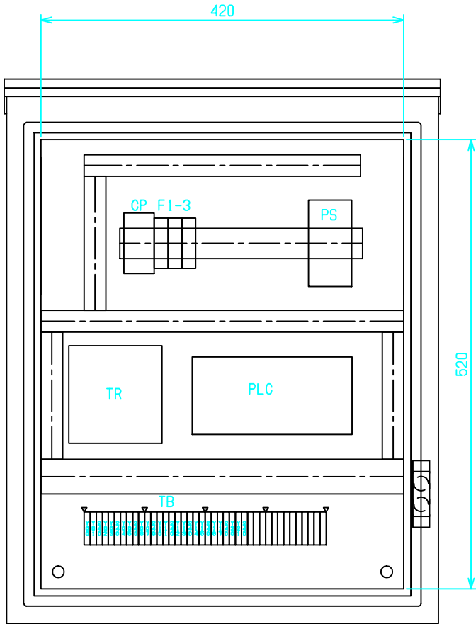
中扉を開けた状態
